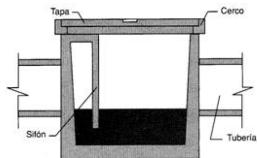
SECCION ARQUETA SIFONICA HV
